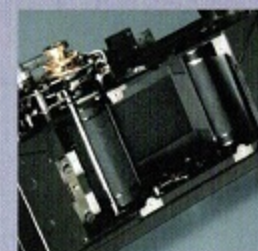
最高速1/1000秒の横走り ゴム引き布幕式 フォーカルプレーンシャッター。
